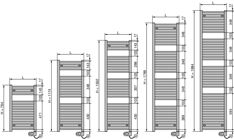
VUE FRONTALE
