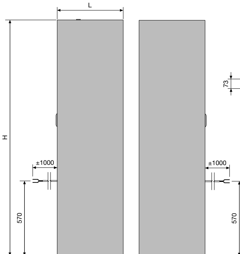
Vue frontale
