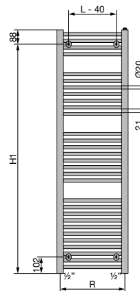
VUE ARRIÈRE
