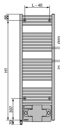
VUE ARRIÈRE
