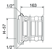
Type 33 Zijaanzicht
