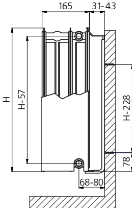
type 33
