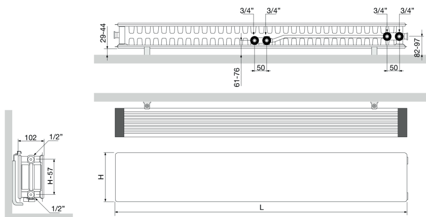
Type 22 Zijaanzicht
