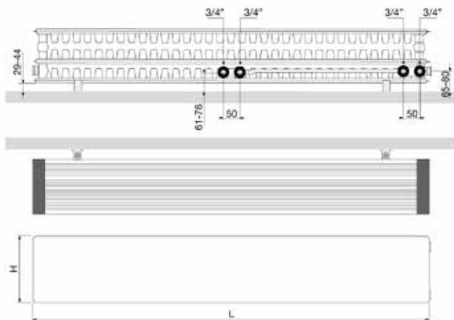
Type 33 Onderaanzicht
