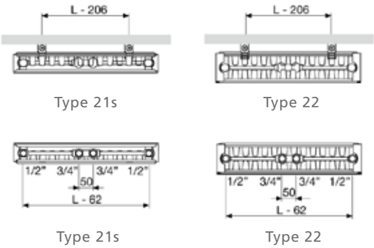
ONDERAANZICHT
