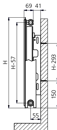
type 11
