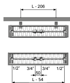
Onderaanzicht
