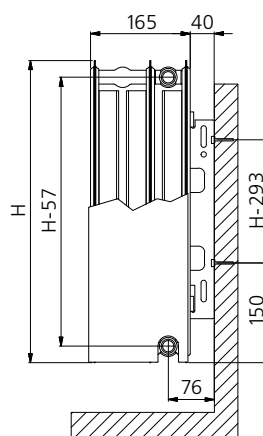
type 33
