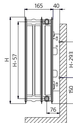
type 33
