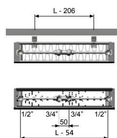
Onderaanzicht
