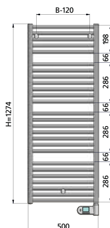
Vooraanzicht
