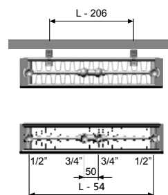
Onderaanzicht
