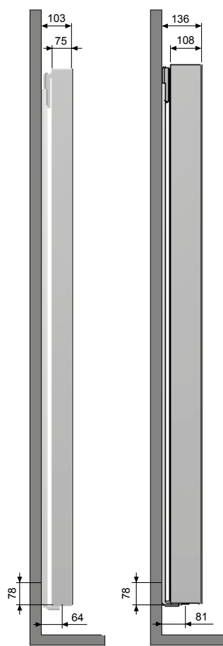
Zijaanzicht
