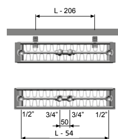
Onderaanzicht
